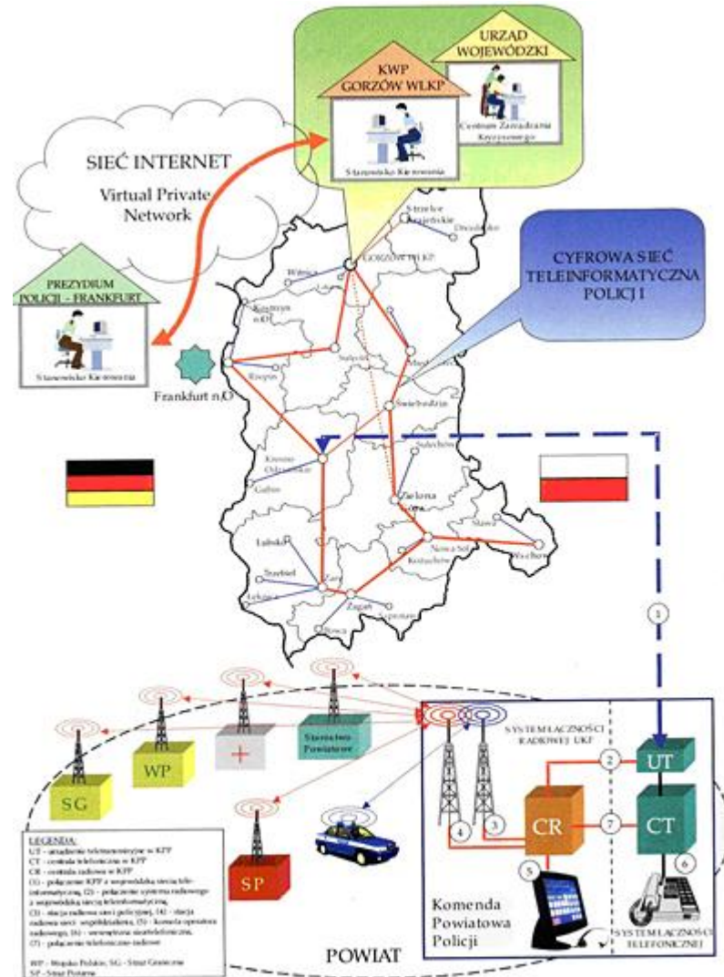
Rys. 1. Poglądowy schemat integracji systemu łączności przewodowej i radiowej Policji oraz sposobu współdziałania z innymi służbami w wymiarze powiatowym, wojewódzkim i transgranicznym.
